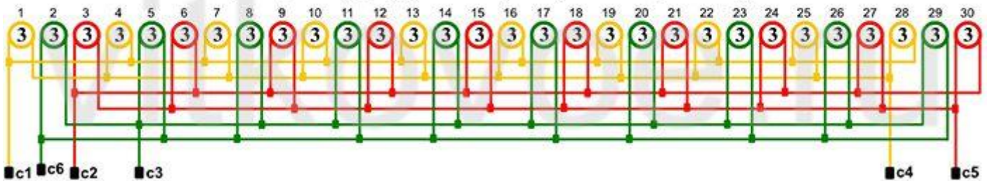
2p=10 ; Z=90 ; q=3 ; y=7 или 8 ; a=10 ; обмотка равнокатушечная
