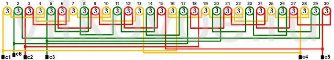
2p=10 ; Z=90 ; q=3 ; y=7 или 8 ; a=2 ; обмотка равнокатушечная
