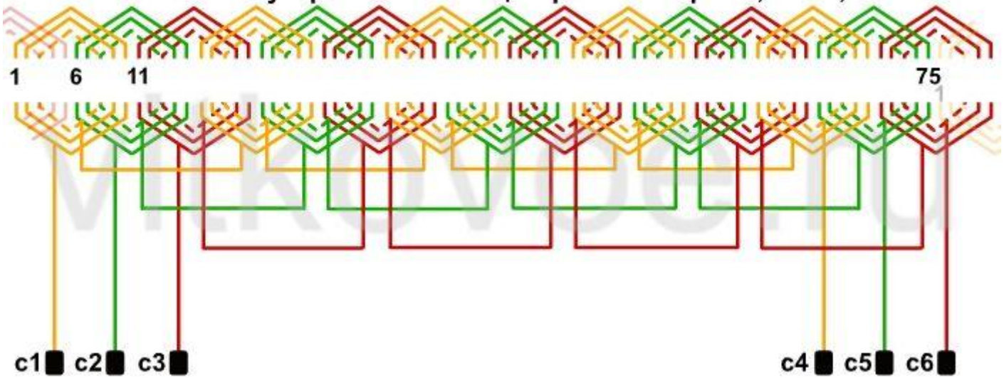
Обмотка полутораслойная концентрическая 2p=10 ; Z=75 ; a=1
