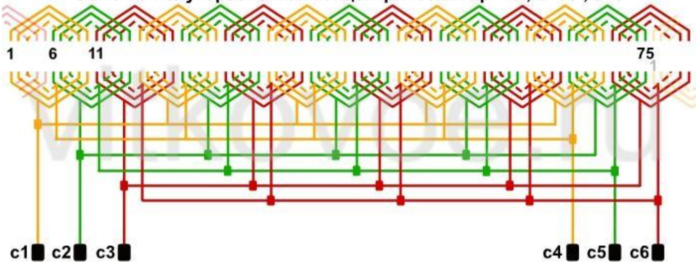
Обмотка полутораслойная концентрическая 2p=10 ; Z=75 ; a=5
