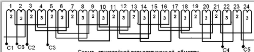
.Схема двухслойной равнокатушечной обмотки: 2p=8, Z=60, q=2 \text{ и } 3, u=1-7, a=1
