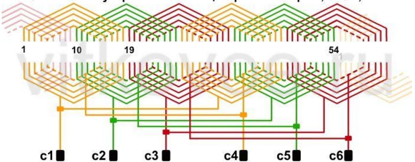
Обмотка полутораслойная концентрическая 2p=4 ; Z=54 ; a=2
