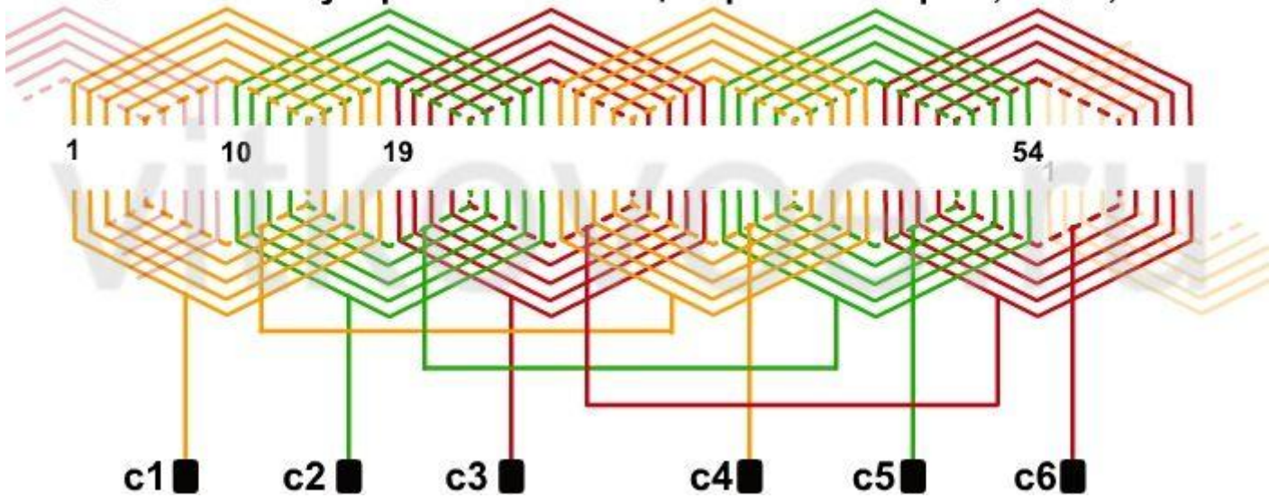
Обмотка полутораслойная концентрическая 2p=4 ; Z=54 ; a=1
