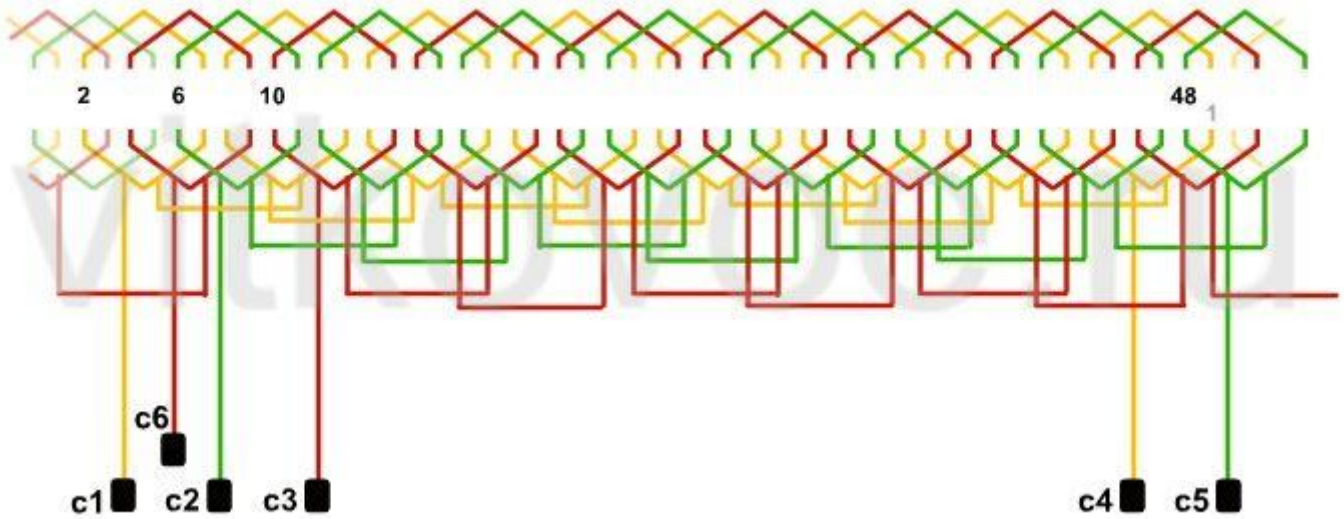
Обмотка однослойная "вразвалку" 2p=8 ; Z=48 ; y=1-6 ; a=1
