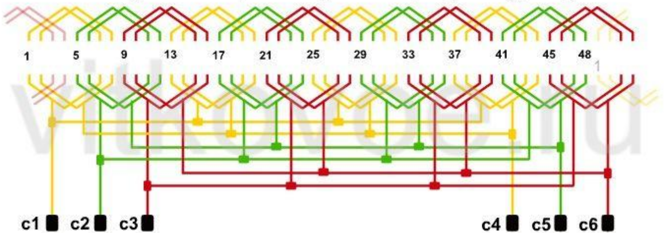
Обмотка однослойная равнокатушечная 2p=8 ; Z=48 ; y=1-7 ; a=4
