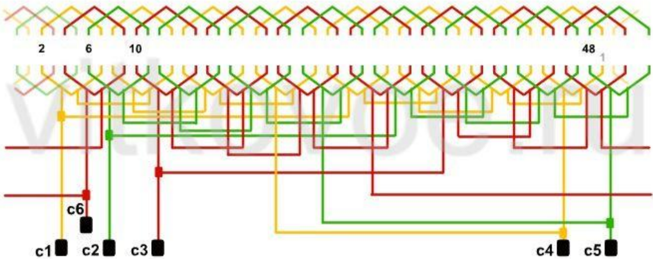
Обмотка однослойная "вразвалку" 2p=8 ; Z=48 ; y=1-6 ; a=2
