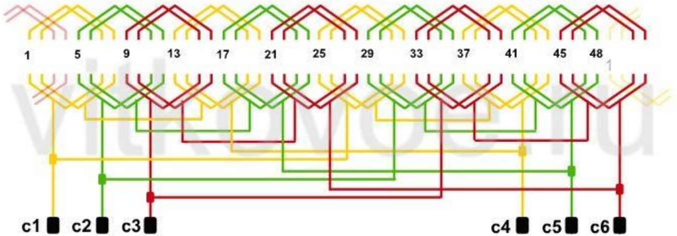
Обмотка однослойная равнокатушечная 2p=8 ; Z=48 ; y=1-7 ; a=2
