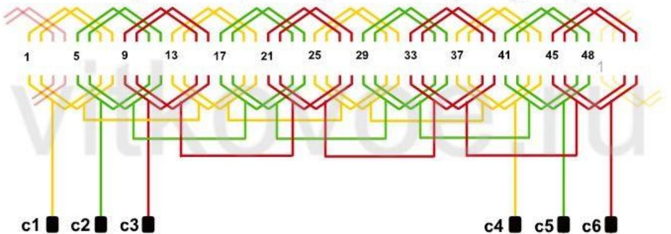
Обмотка однослойная равнокатушечная 2p=8 ; Z=48 ; y=1-7 ; a=1
