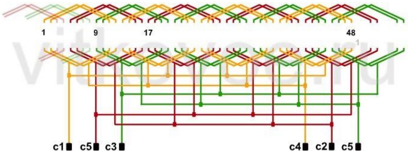
Однослойная равнокатушечная обмотка "вразвалку" 2p=4 ; Z=48 ; y=10 ; a=4
