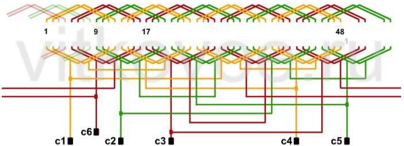
Однослойная равнокатушечная обмотка "вразвалку" 2p=4 ; Z=48 ; y=10 ; a=2
