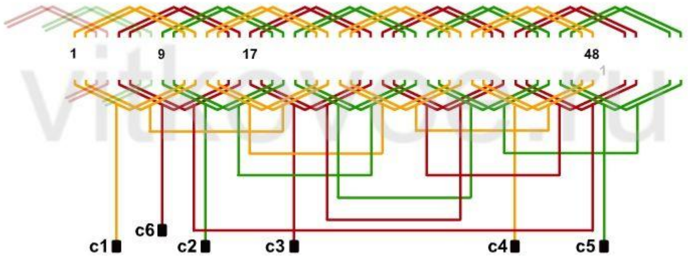
Однослойная равнокатушечная обмотка "вразвалку" 2p=4 ; Z=48 ; y=10 ; a=1
