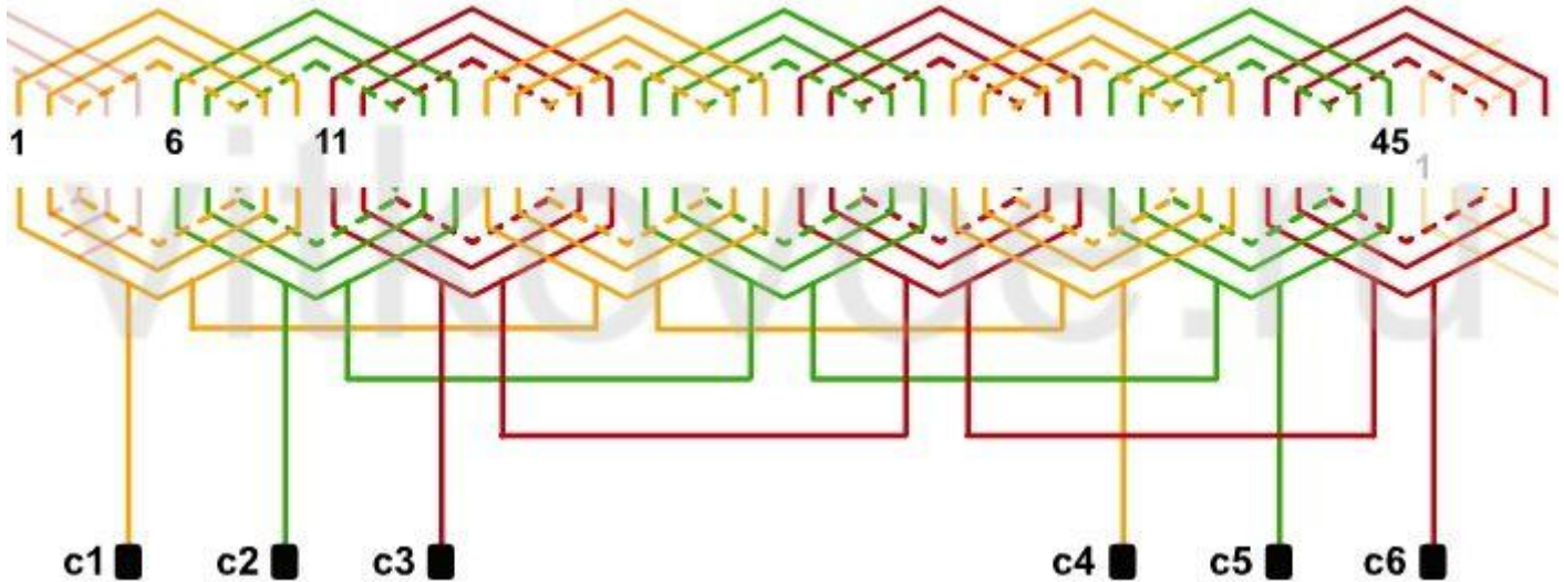
Обмотка полтораслойная концентрическая 2p=6 ; Z=45 ; y=9,7,5 ; a=1
