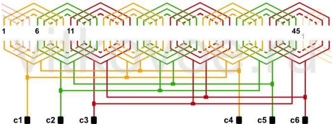
Обмотка полтораслойная концентрическая 2p=6 ; Z=45 ; y=9,7,5 ; a=3
