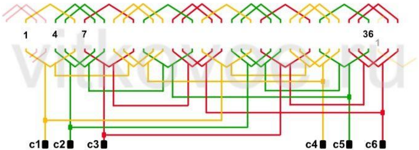
Однослойная обмотка 2p=8 ; Z=36 ; q=1и2 ; y=5,4 ; a=2
