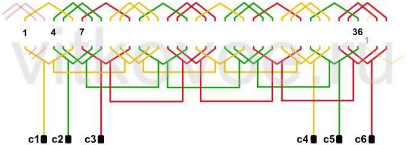
Однослойная обмотка 2p=8 ; Z=36 ; q=1и2 ; y=5,4 ; a=1
