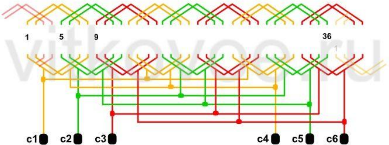
Обмотка однослойная равнокатушечная 2p=6 ; Z=36 ; y=6 ; a=3
