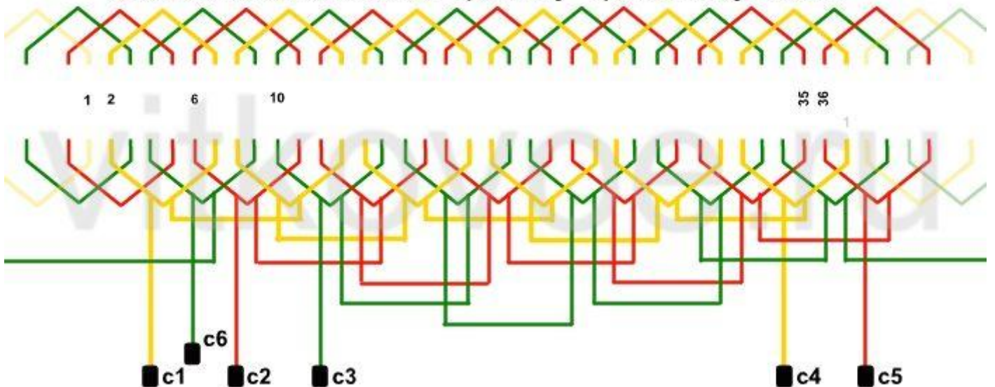
Схема однослойной обмотки "вразвалку" 2p=6 ; Z=36 ; y=1-6 ; a=1
