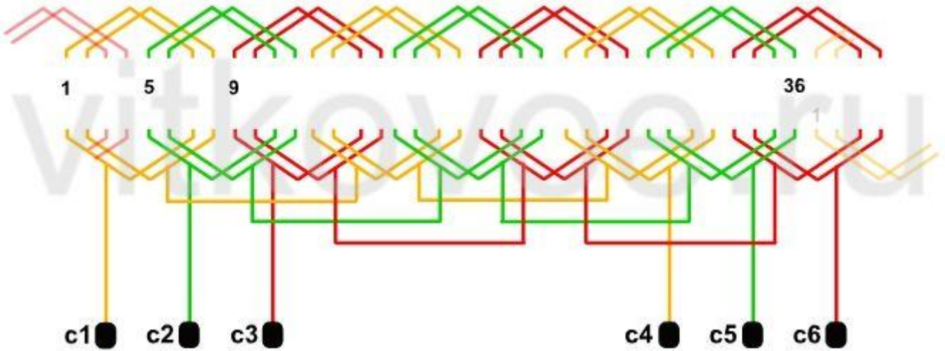
Обмотка однослойная равнокатушечная 2p=6 ; Z=36 ; y=6 ; a=1
